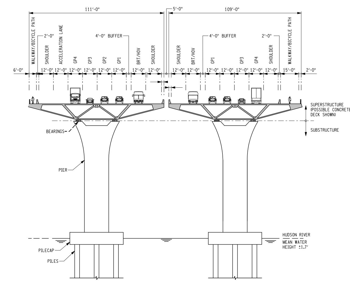
SECTION 6 AT STA. 995+00 SCALE: 1"=20'-0"
